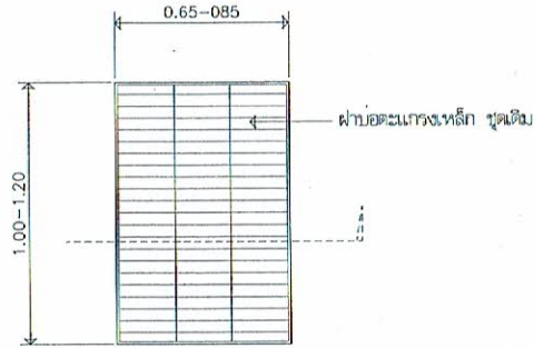
ขยายฝาครอบน้ำ MH มาตราส่วน 1 : 25
