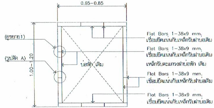
แปลนเหล็กท่อนฝาครอบน้ำ MH มาตราส่วน 1 : 25
