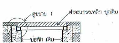
รูปตัดฝาครอบน้ำ มาตราส่วน 1 : 25
