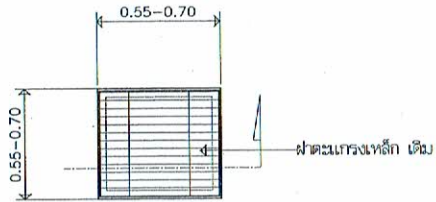
ขยายฝาครอบน้ำ มาตราส่วน 1 : 25
