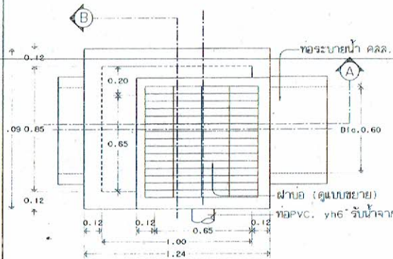
แปลนระบบระบายน้ำในผิวจราจร SCALE 1:25
