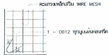
ขยายการเสริมเหล็กกันร้าว
