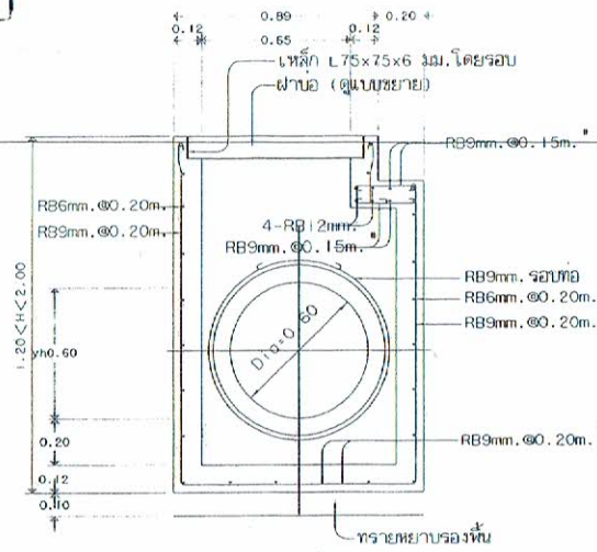
รูปตัด B-B SCALE 1:25
