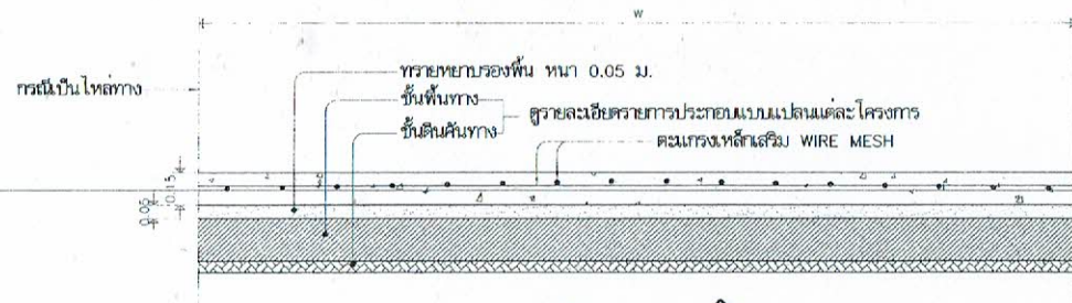
รูปตัด SCALE 1:25
