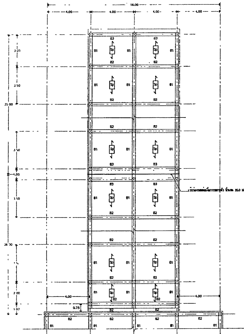
แปลนคานรับเสาเข็มสะพานช่วงทางเดิน มาตราส่วน 1:100
