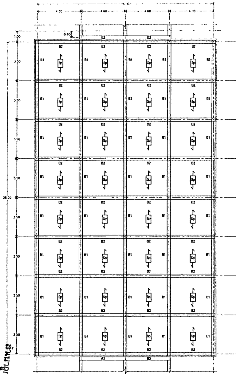
แปลน โครงสร้างพื้นและคานช่วงคานภายนอกประสงค์ มาตราส่วน 1:100
