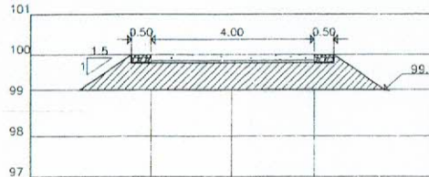
A=4.45 STA.0+200.00 Scale 1:100
