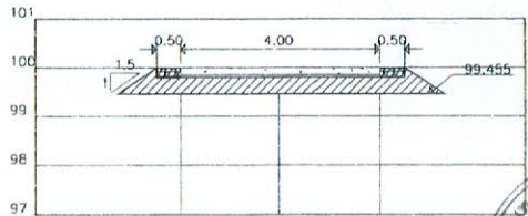
A=2.17 STA.0+100.00 Scale 1:100
