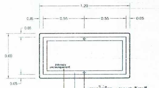
ป้ายโครงการงานก่อสร้าง SCALE 1:20
