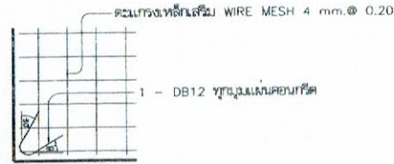
ขยายการเสริมเหล็กกันร้าว SCALE 1:50
