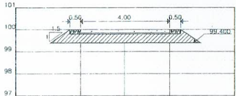
A=2.57 STA.0+075.00 Scale 1:100
