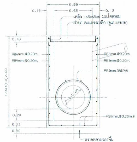
รูปตัด B SCALE 1:25
