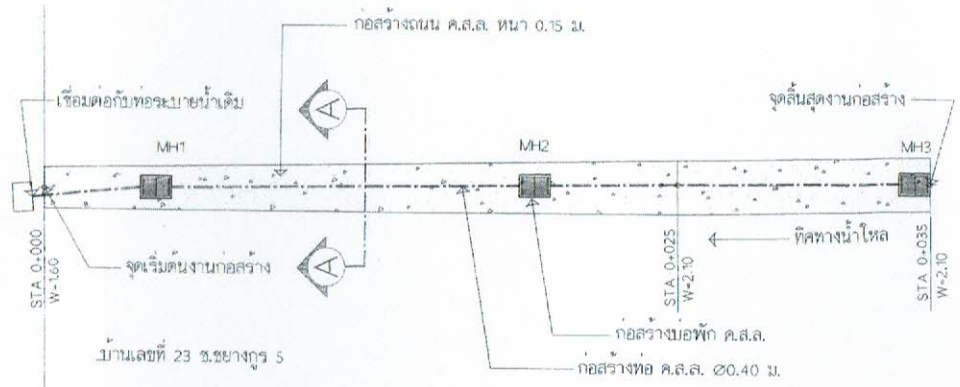
แปลนก่อสร้างถนน ค.ส.ล. พร้อมท่อระบายน้ำ มาตราส่วน 1:200
