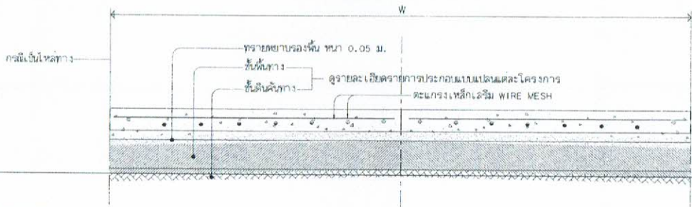
รูปตัด SCALE 1:25
