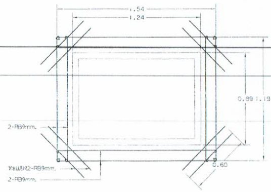
แปลนฝาปิดคสล. และ เหล็กเสริมรอบขอบคสล. SCALE 1:25
