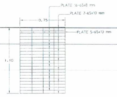
ขยายฝาปิดคสล. และ เหล็กเสริมรอบขอบคสล. สำหรับขอบคสล. 0.40 ม. SCALE 1:25
