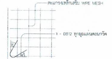
ขยายการเสริมเหล็กกั้นมุม SCALE 1:50
