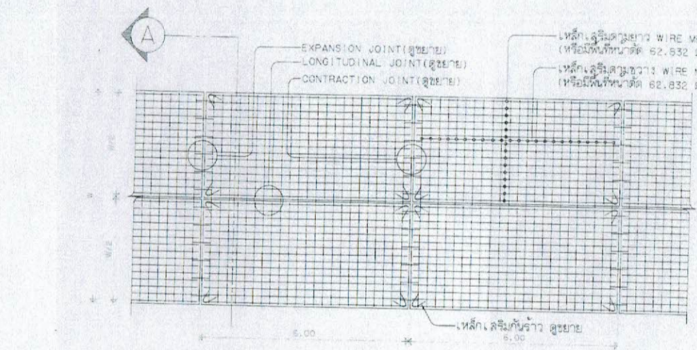
แปลนถนน ค.ล.ล. (หนา 0.15 ม.) SCALE 1:100
