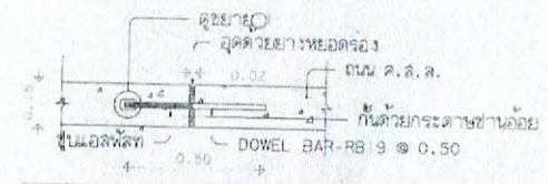
EXPANSION JOINT 1:20 (ทุกระยะไม่เกิน 60.00 ม.)
