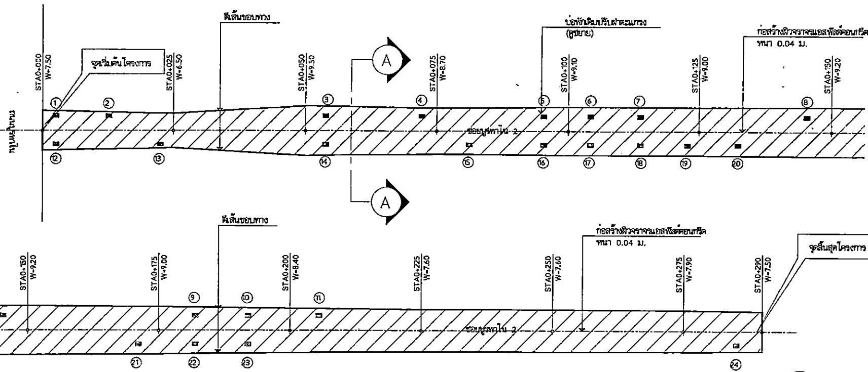
แบบรูปแอสฟัลต์คอนกรีต SCALE 1:500
