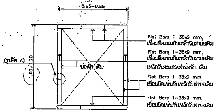
แปลนเหล็กทูนฝาปิดเหล็ก MH มาตราส่วน 1 : 25
