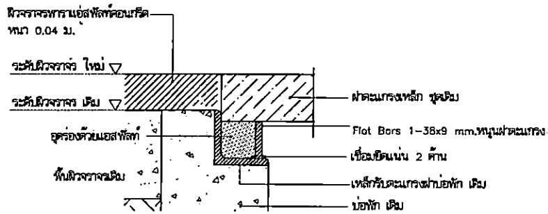
ขยาย 1 มาตราส่วน 1 : 5
