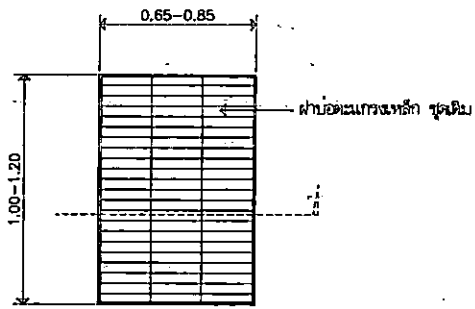
ขยายฝาปิดเหล็ก MH มาตราส่วน 1 : 25
