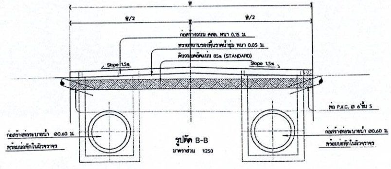
ค.ส.ล. แผนก่อสร้างถนน ค.ส.ล. พร้อมท่อชะลอน้ำ หมายเลข 24 มกราคม 1750
