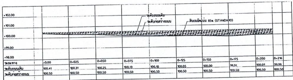
รูปตัดตามยาว ซอยชายงูกร 22 แนวตั้ง ๕100 แนวนอน ๕1000
