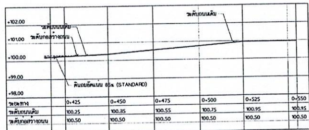
รูปตัดตามยาว ซอยชายงูกร 24 แนวตั้ง ๕100 แนวนอน ๕1000
