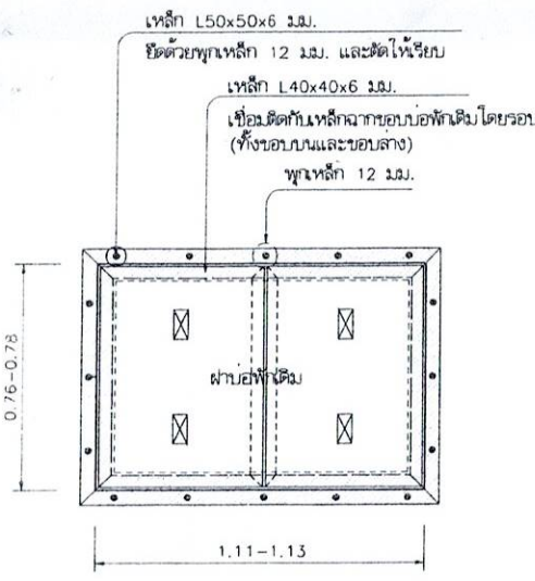
แปลนบอพัทัก 1:20
