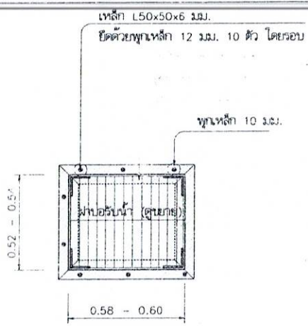
แปลนบออร์รับน้ำ 1:20
