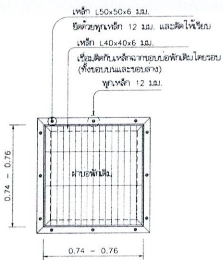
แปลนบอพัทัก 1:20
