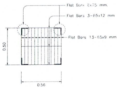
ขยายฝ้าออร์รับน้ำ 1:20
