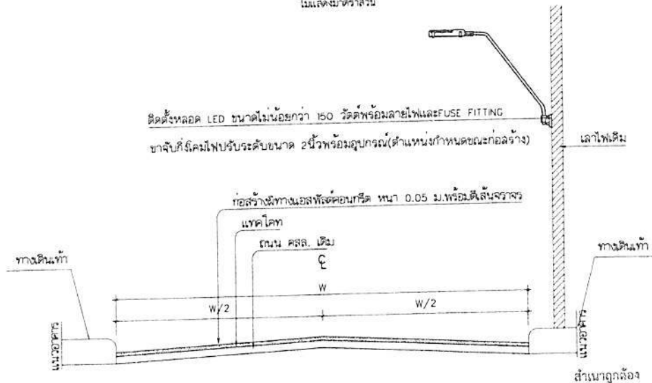
รูปตัด A-A non scale
