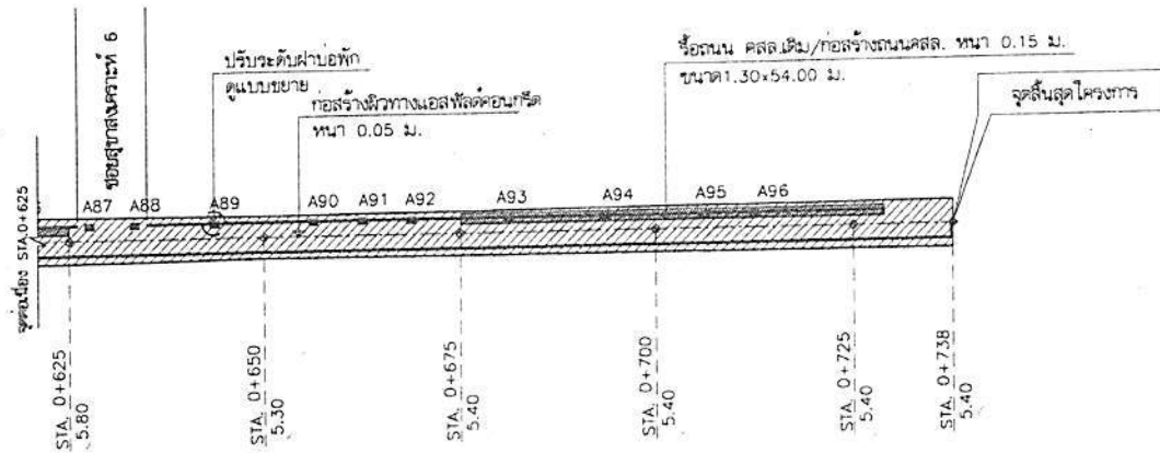
แปลนปูแอสฟัลต์คอนกรีตใต้เส้นจราจร SCALE 1:750
