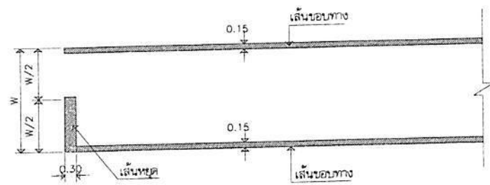
ขยายงานใต้เส้นจราจร ไม่แสดงขนาดส่วน
