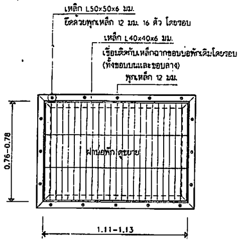
แบบขยายฝาม่อพัก C มาตราส่วน 1:20
