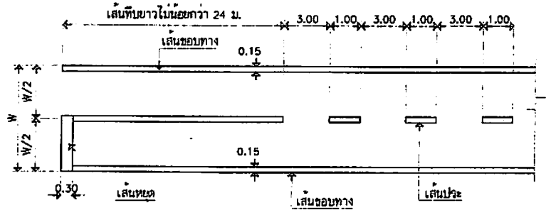
ขยายงานติดตั้งเสาจราจร ไม่แสดงขนาดส่วน
