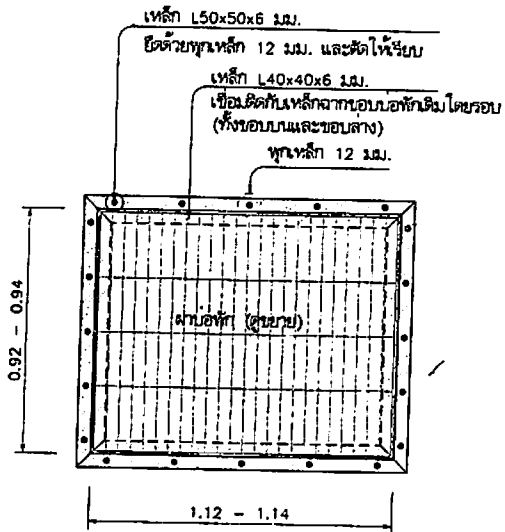
แบบสนบ่อพัก J 1:20
