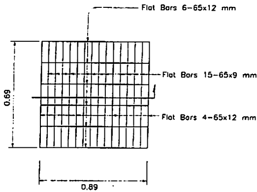
ขยายฝ้าบ่อพัก H 1:20
