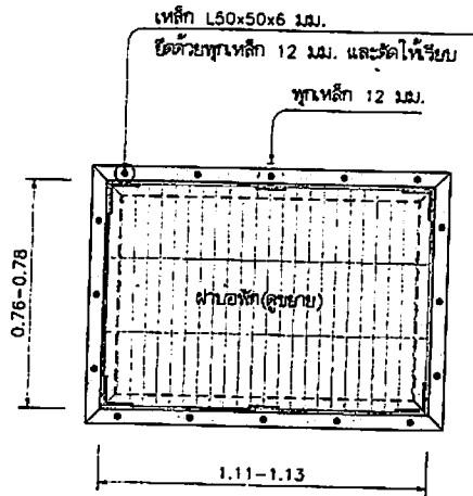
แปลนบ่อพัก D 1:20
