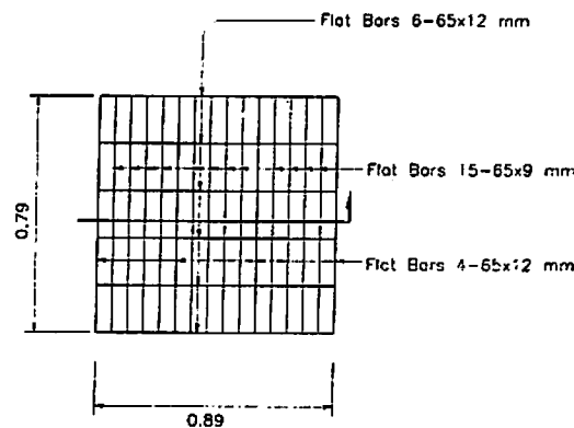
ขยายฝ้าบ่อพัก I 1:20
