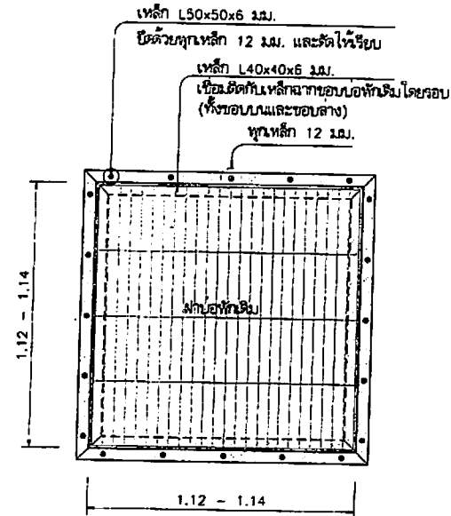
แบบสนบ่อพัก L 1:20
