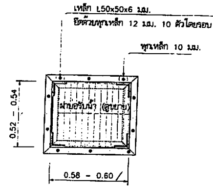
แปลนบ่อรับน้ำ G 1:20
