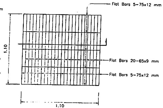
ขยายฝ้านบ่อพัก L 1:20
