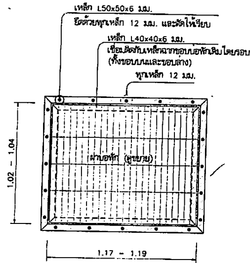
แบบสนบ่อพัก K 1:20
