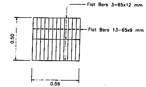
ขยายฝ่าบ่อรับน้ำ F 1:20
