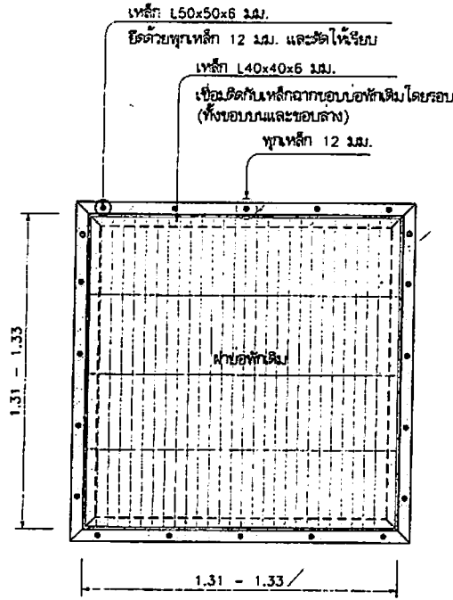
แปลนบ่อพัก M 1:20
