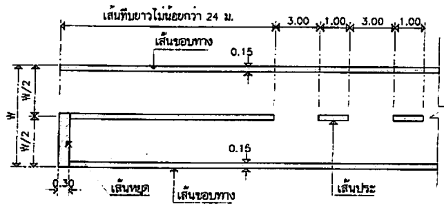
ขยงานตีเส้นจราจร ไม่แสดงมาตราส่วน
