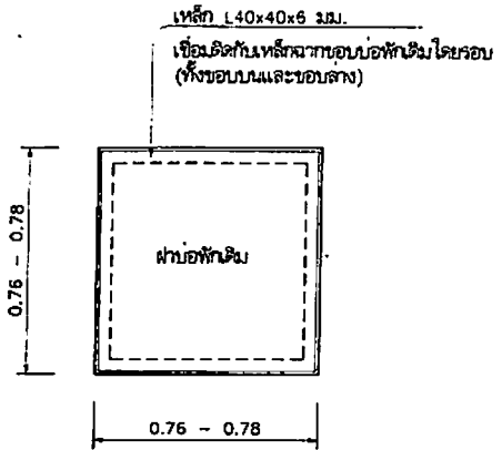
แปลนบ่อพัก A 1:20
