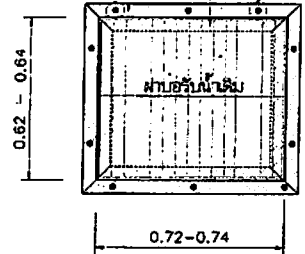
แปลนบ่อพัก A 1:20
