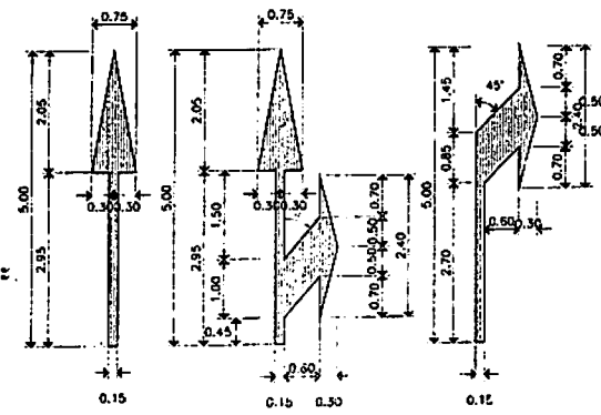
มาตรฐานเครื่องหมายลูกศรบนผิวทาง
