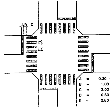
มาตรฐานสีสว่างคนข้ามที่ทางแยก
