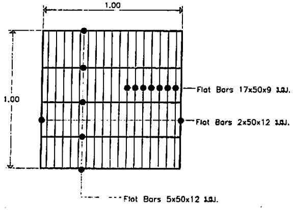
แบบขยายฝ้าปิดตะแกรง C 1:20
