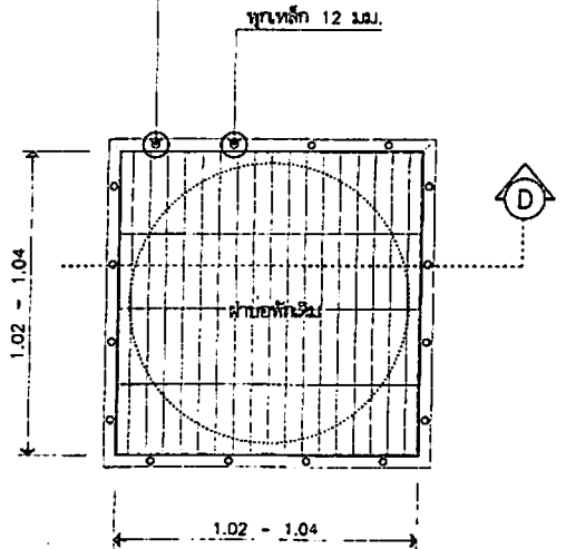
แปลนบ่อพัก C 1:20
