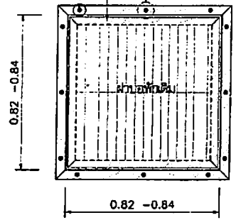
แปลนบ่อพัก B 1:20
