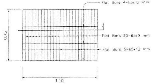
ขยายฝ้าบ่อพัก B 1:20
