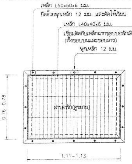
แปลนบ่อพัก B 1:20
