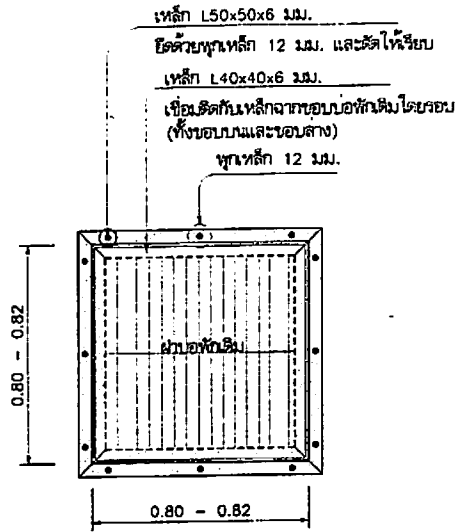
แปลนบ่อพัก A 1:20
