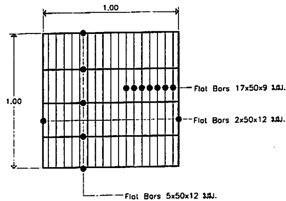
แบบขยายฝ้าปิดตะแกรง B 1:20
