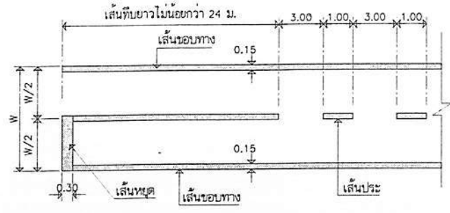
ขยายงานเดินเส้นจราจร ไม่แสดงมาตราส่วน
