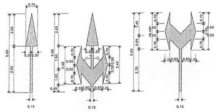
มาตรฐานเครื่องหมายลูกศรบนผิวทาง
