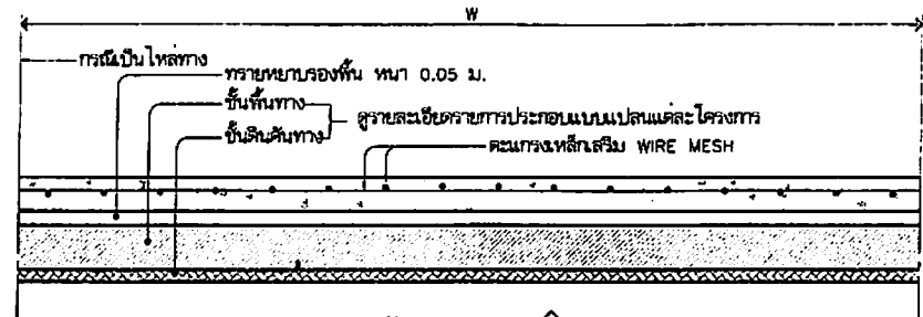
รูปตัด SCALE 1:25
