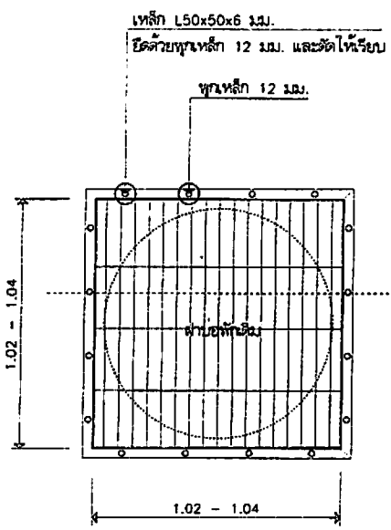
แปลนบ่อพัก H 1:20
