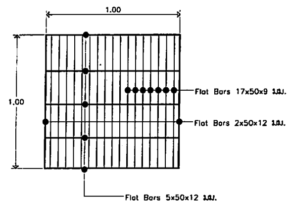
แบบขยายฝาปิดตะแกรง H 1:20
