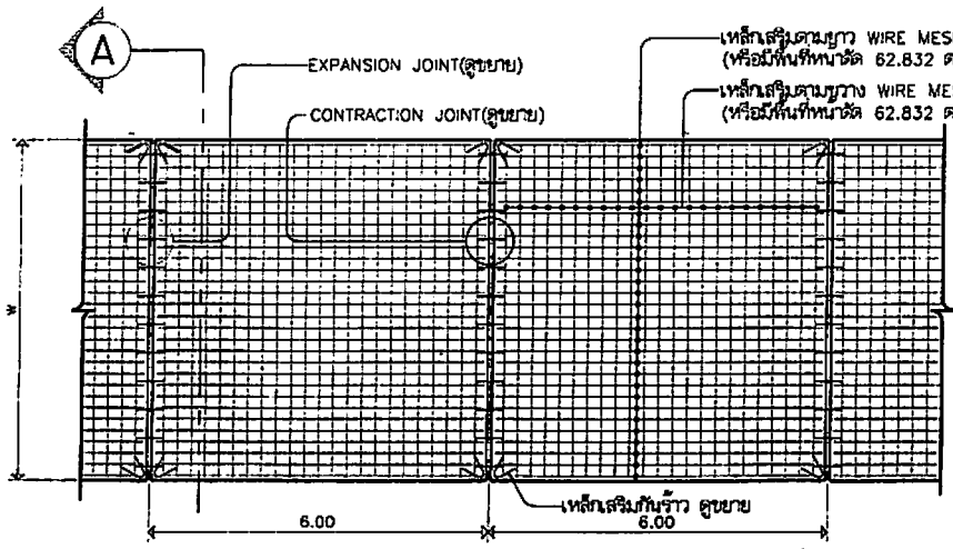
แปลนถนน ค.ส.ล. (หนา 0.15 ม.) SCALE 1:100
