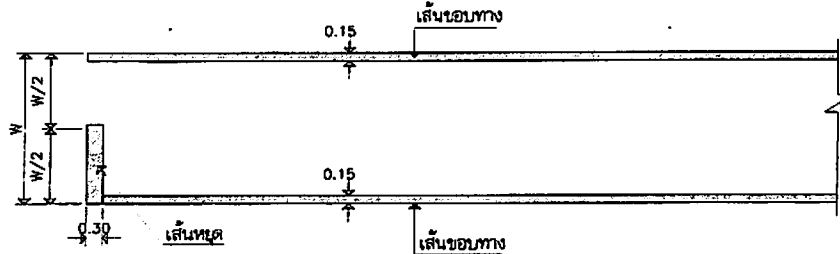
ขยายงานตีเส้นจราจร โมดูลขนาดบางส่วน
