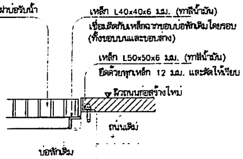
รูปตัด 1:10
