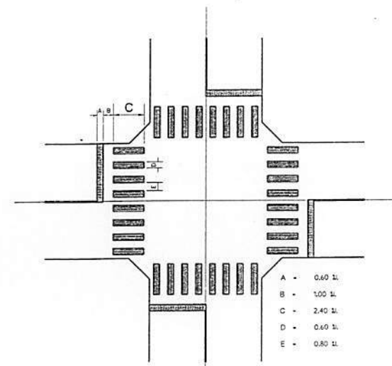
มาตรฐานเส้นทางคนข้ามที่ทางแยก SCALE : 250
