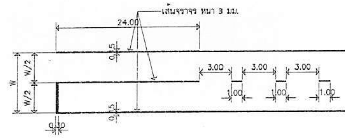
มาตรฐานเส้นแบ่งช่องจราจร SCALE : 250 สำหรับรถสองล้อ
