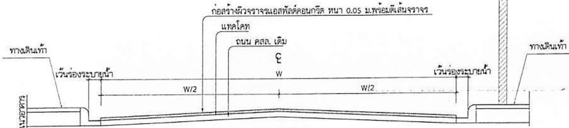
รูปตัด A-A non scale
