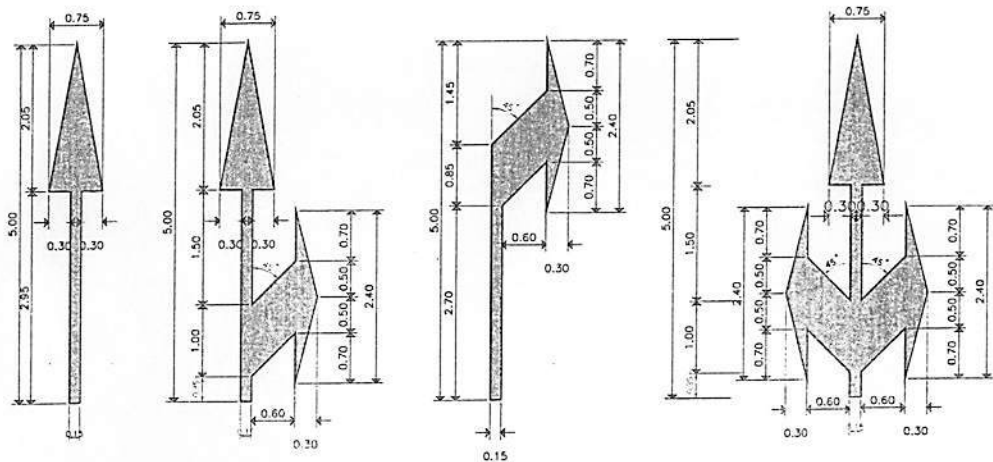
มาตรฐานเครื่องหมายลูกศรบนผิวทาง SCALE : 50
