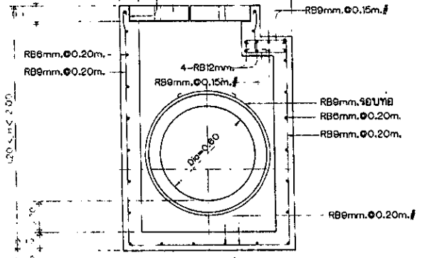
รูปตัด B SCALE 1:25
