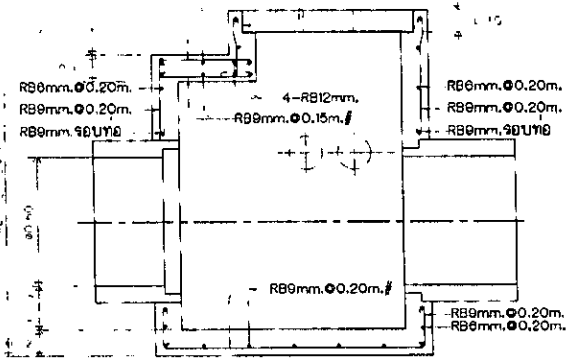
รูปตัด A SCALE 1:25
