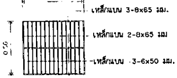
รูปขยายฝ้าตะแกรงเหล็กบ่อรับน้ำ SCALE 1:25
