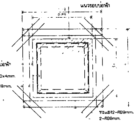
แบบขยายเหล็กเสริมรอบบ่อพัก SCALE 1:25
