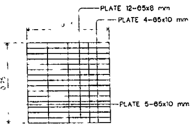
แบบขยายฝ้าตะแกรงเหล็ก SCALE 1:25
