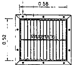
ขยายการยกผ่านตะแกรงเหล็กบ่อรับน้ำ 1:20
