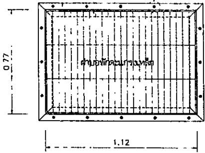
ขยายการยกผ่านบ่อพักตะแกรงเหล็ก 1:20
