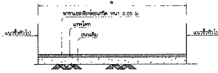
รูปตัด ทัวไป
