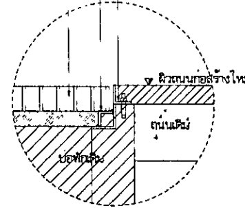
ขยายการยกผ่านบ่อ 1:10
