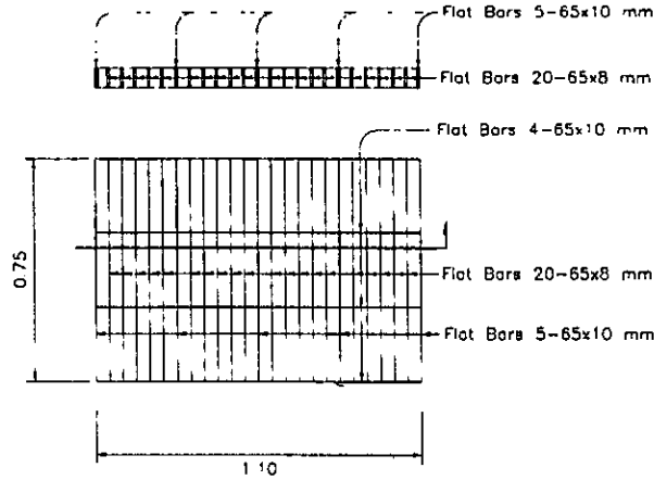
ขยายผ่านบ่อพักตะแกรงเหล็ก 1:20
