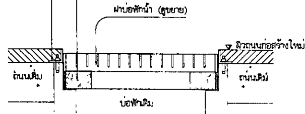
ขยายการยกผ่านบ่อรับน้ำ 1:10
