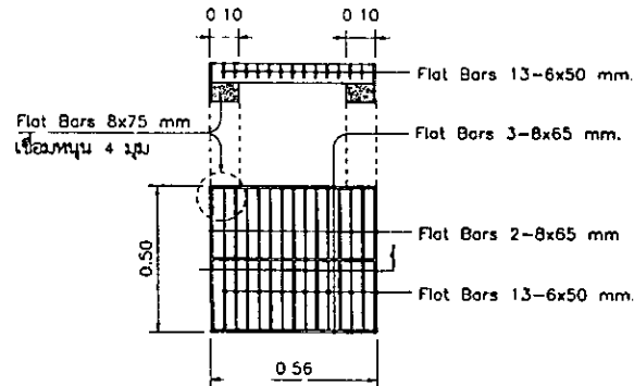
ขยายผ่านตะแกรงเหล็กบ่อรับน้ำ 1:20
