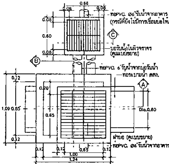
แปลนระบบระบายน้ำในครัวจาง SCALE 1:25
