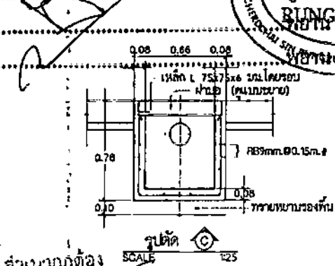
รูปตัด C SCALE 1:25
