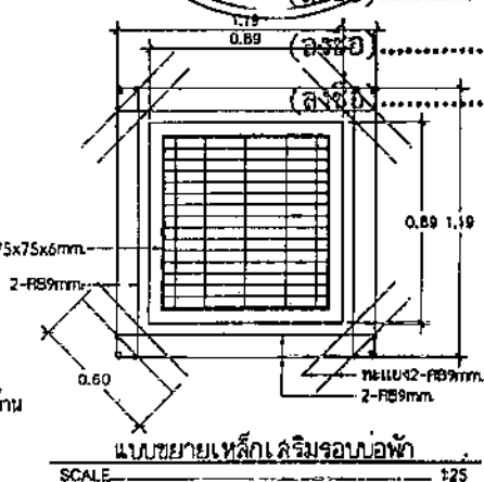
แปลนขยายเหล็กเสริมรอบบ่อพัก SCALE 1:25
