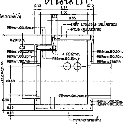
รูปตัด A SCALE 1:25
