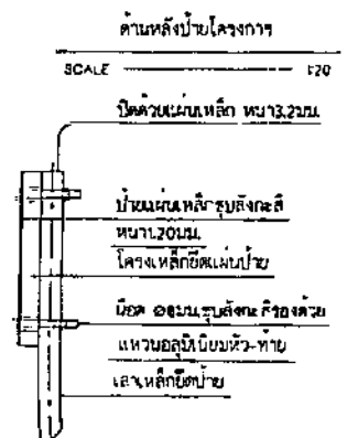
การติดตั้งป้ายโครงการ
