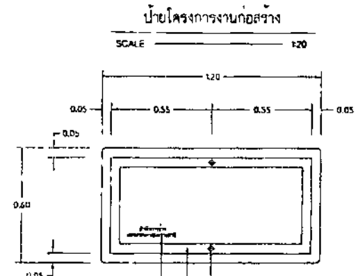
ป้ายโครงการงานก่อสร้าง SCALE 1:20 ชื่อหน่วยงานผู้ดำเนินการก่อสร้าง ตัวอักษรสีดำสูง 0.03ม. เจาะรูใส่นอต อกรรมชุบสังกะสี หรือบนีส อกรรมชุบสังกะสี โครงเหล็กถากขนาด 1.1 x 2.2 ม. เขียนโดยรอบ ทาสีกันสนิม 2 ครั้งแล้วทาสีขาวครึ่ง
