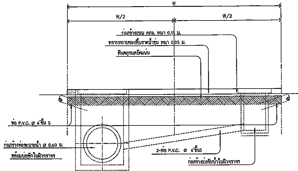
รูปตัด A-A มาตราส่วน 1:250
