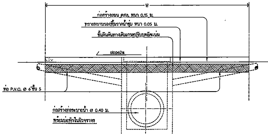
รูปตัด B-B มาตราส่วน 1:200
