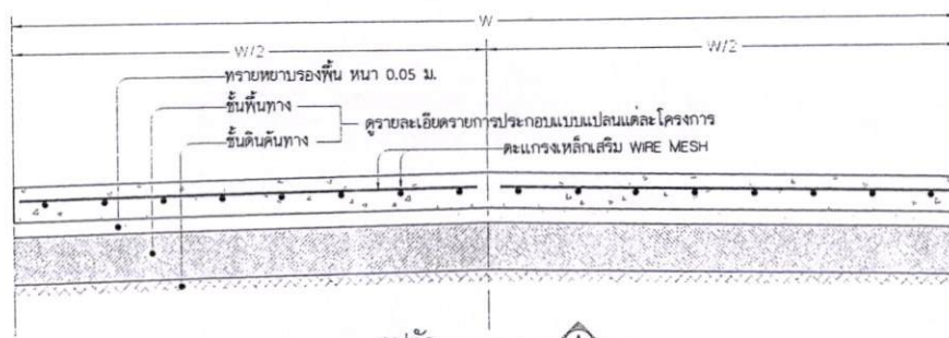
รูปตัด A-A SCALE 1:25
