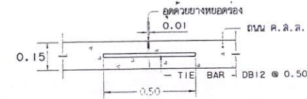
LONGITUDINAL JOINT 1:20
