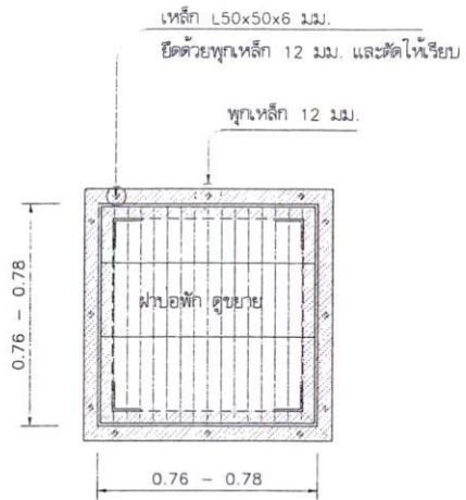
แปลนบ่อพัก C 1:20
