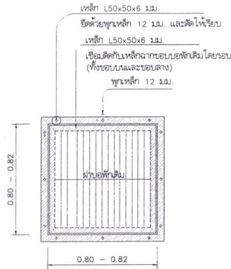
แปลนบ่อพัก A 1:20 ฝาบ่อพักเดิมขนาด 0.78 x 0.78 ม.
