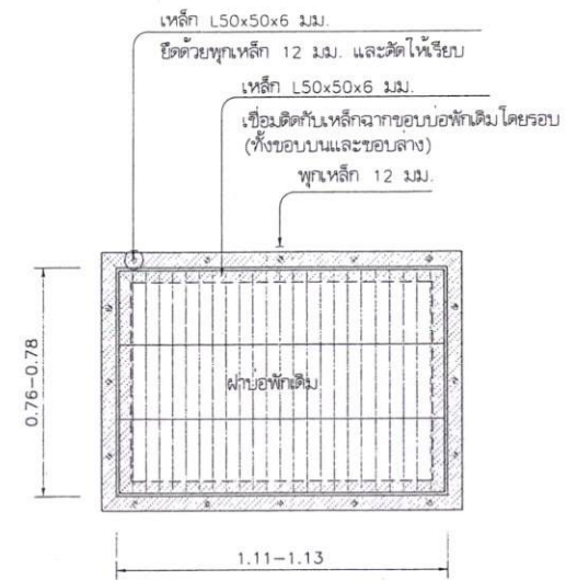
แปลนบ่อพัก B 1:20 ฝาบ่อพักเดิมขนาด 0.75 x 1.10 ม.
