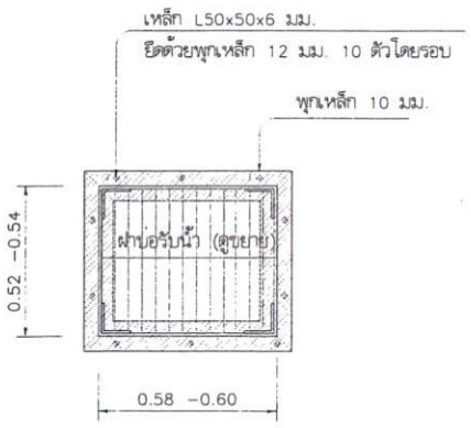
แปลนบ่อรับน้ำ D 1:20
