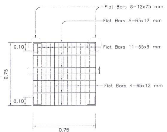
ขยายผ้าอพัก C 1:20
