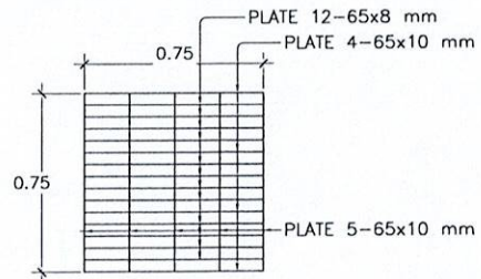
แบบขยายฟลักซ์ SCALE 1:25
