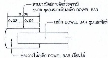
รูปตัด I-I SCALE 1:2.5
