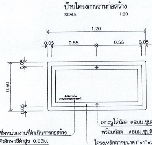
ด้านหลังบ้ายโครงการ SCALE 1:20
