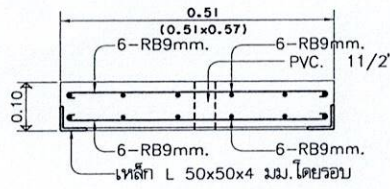
รูปตัดขยายฟลักซ์รับน้ำ คสล. SCALE 1:10
