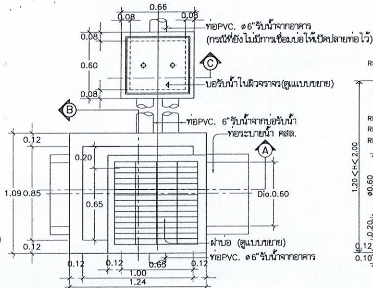
แปลนระบบระบายน้ำในผิวจากราง SCALE 1:25
