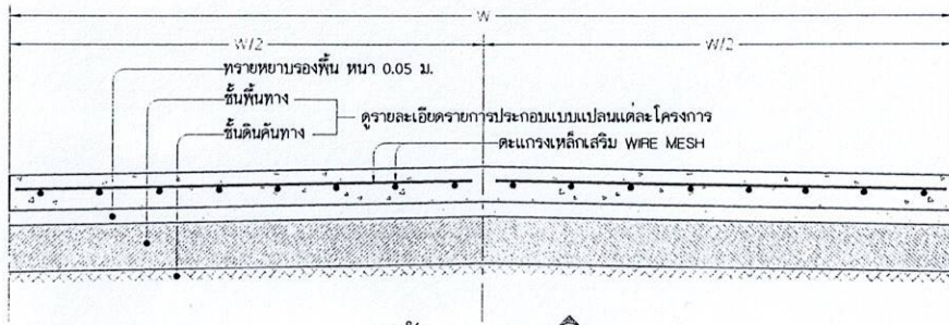
รูปตัด A-A SCALE 1:25
