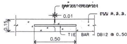
LONGITUDINAL JOINT 1:20
