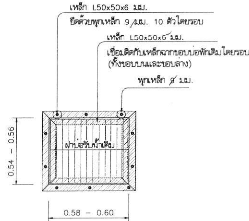
แปลนบ่อรับน้ำ C 1:20
