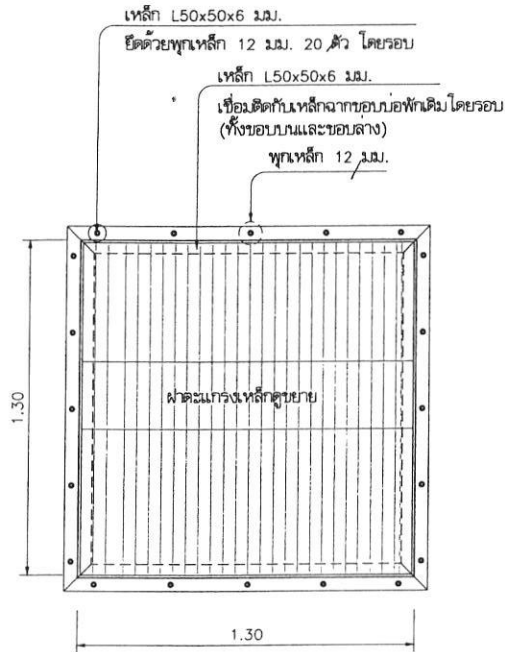
แปลนบ่อพัก B 1:20
