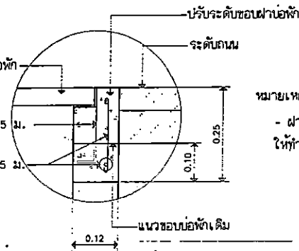
ขยายผิวบ่อรับน้ำ B 1:20
