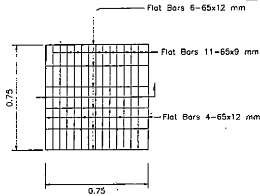
ขยายผิวบ่อพัก A 1:20
