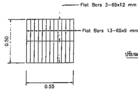
ขยายผิวบ่อรับน้ำ B 1:20
