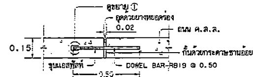
EXPANSION JOINT 1:20 (ทุกระยะ ไม่นเกิน 60.00 ม.)
