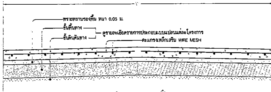
รูปตัด B SCALE 1:25
