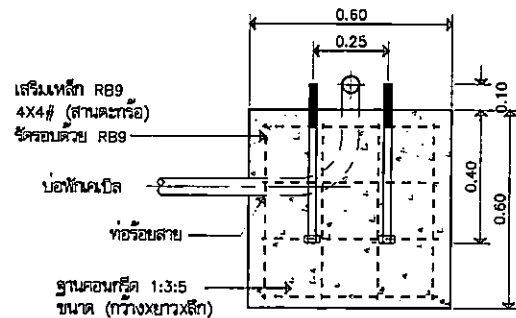
รูปตัดฐานคอนกรีต มาตราส่วน 1:25
