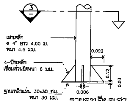
รายละเอียดเสาหลัก มาตราส่วน 1:12.5
