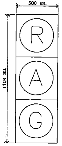
แบบขยายโคมไฟ LED 3 ดวง
