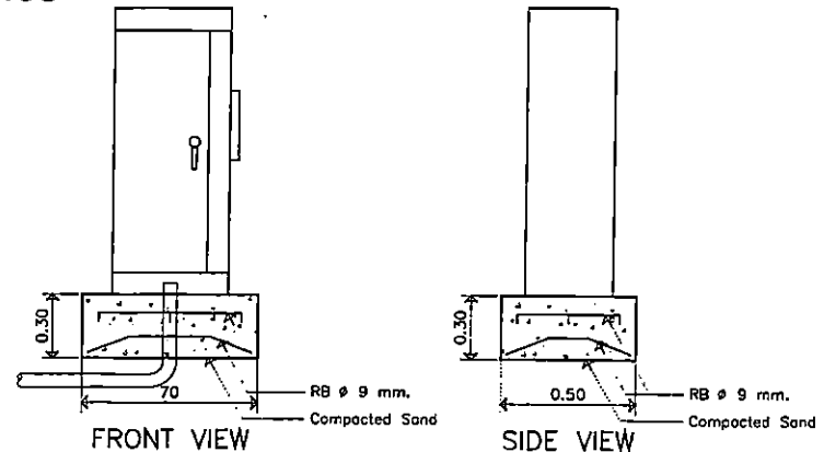
ตู้เครื่องควบคุมสัญญาณไฟจราจร
