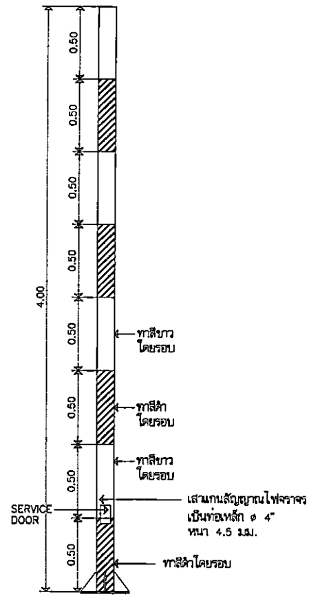
แบบเสาสัญญาณไฟจราจรแบบที่ 2 มาตราส่วน 1:25
