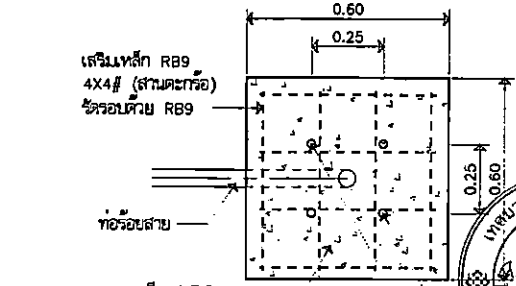
แบบฐานคอนกรีต มาตราส่วน 1:25
