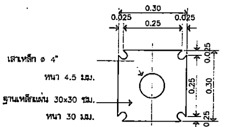
แบบฐานโคนเสา มาตราส่วน 1:12.5
