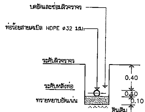
รูปตัด A - A รูปตัดขยายงานลงสายเคเบิล
